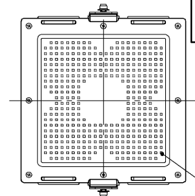
器具取付けボルトを使用した場合の器具内寸法 ※A寸法は、50mm以下にしてください。
