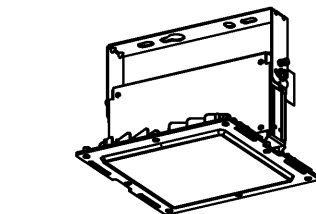
器具取付けボルトを使用した場合の器具内寸法 ※A寸法は、50mm以下にしてください。
