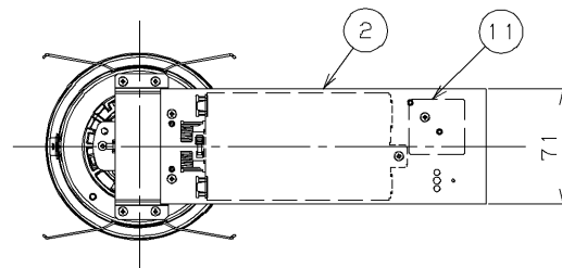
埋込み寸法 取付け可能天井厚: 3mm~25mm
