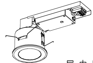
LEDユニット側コネクタと本体側コネクタを接続します。
