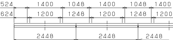
直付け連結使用例
