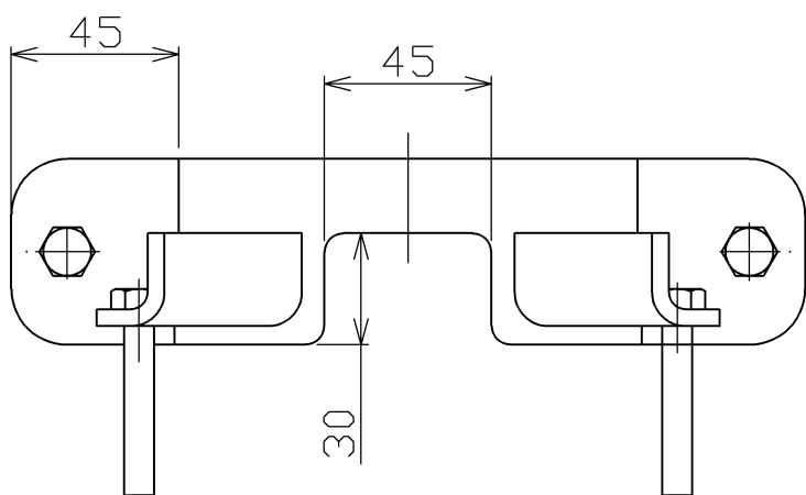
A矢視図
