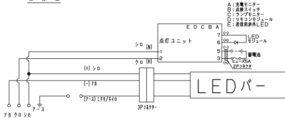
結線図
