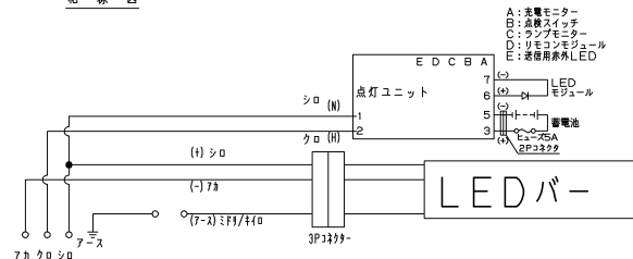
結 線 図
