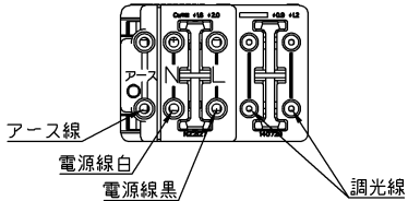
電線差込図
