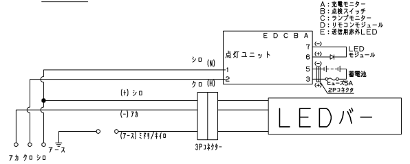
結線図
