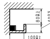
&lt;壁取付の場合&gt;
