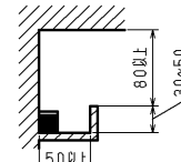
&lt;床置取付の場合&gt;
