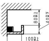
＜壁取付の場合＞
