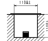
＜密閉床置取付の場合＞
