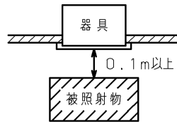
埋込み寸法
