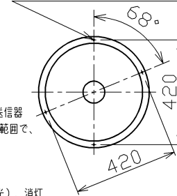
取付けピッチ寸法図 4-φ4.5木ねじ用K.○
