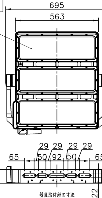
器具取付部の寸法
