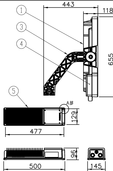
図1 器具の取付と可動範囲
