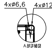
A部詳細図
