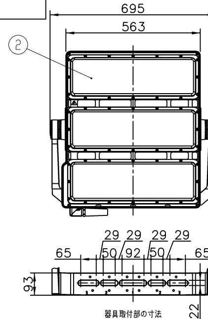
器具取付部の寸法
