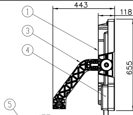
図1 器具の取付と可動範囲
