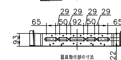
器具取付部の寸法
