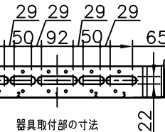
器具取付部の寸法
