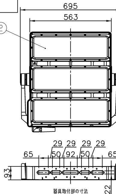
器具取付部の寸法
