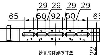
器具取付部の寸法
