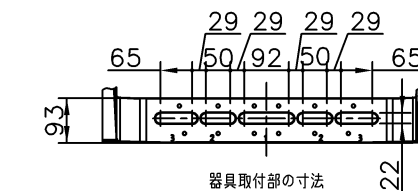
器具取付部の寸法
