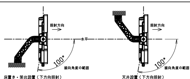
図1 器具の取付と可動範囲
