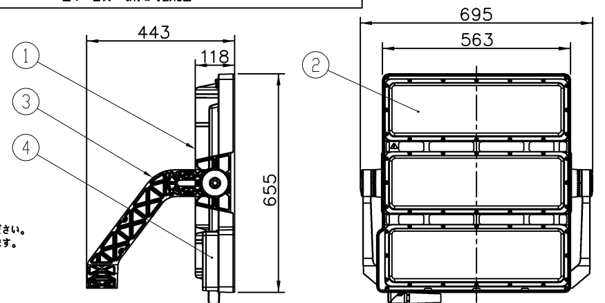
図1 器具の取付と可動範囲
