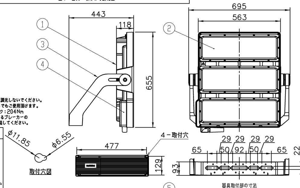
器具取付部の寸法
