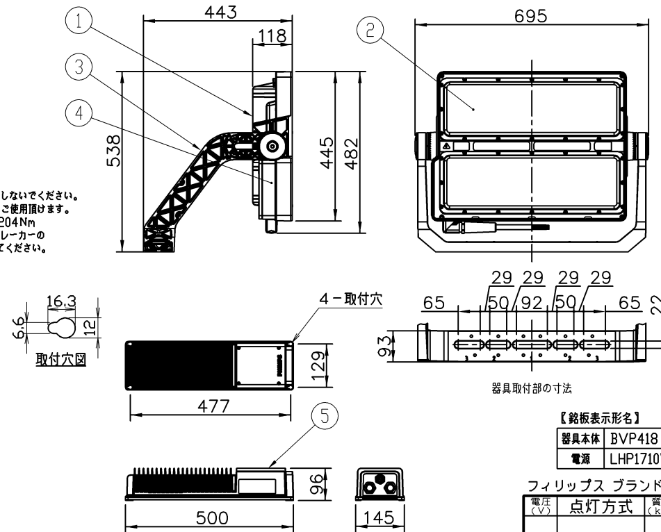
図1 器具の取付と可動範囲
