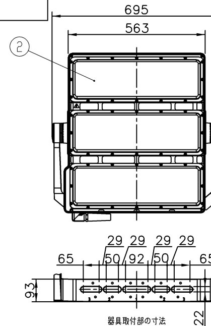
器具取付部の寸法
