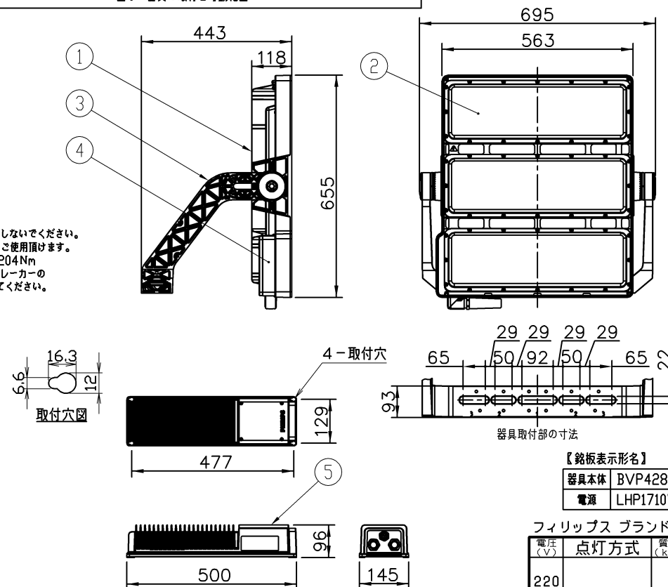
図1 器具の取付と可動範囲
