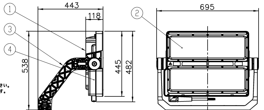
図1 器具の取付と可動範囲
