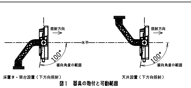
図1 器具の取付と可動範囲
