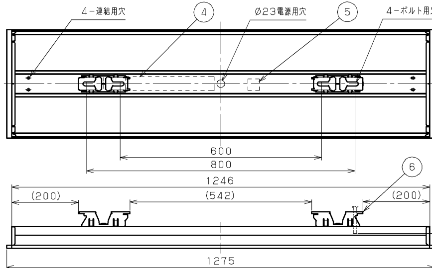
N連結の場合 1275×N-20 埋込み穴寸法
