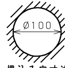
埋込み寸法 取り付け可能な天井厚：5 mm~25 mm
