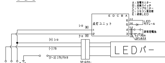
結線図
