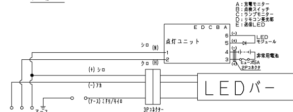
結線図
