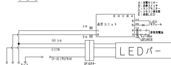
結 線 図
