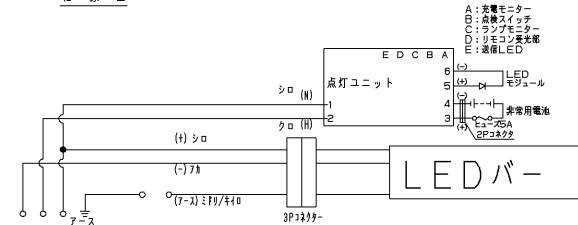
結線図
