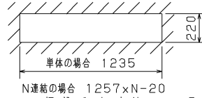
単体の場合 1235 N連結の場合 1257×N-20 埋込み穴寸法
