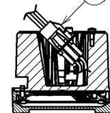
LEDユニット側コネクタと 本体側コネクタを接続します。
