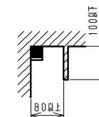
&lt;直付の場合&gt;
