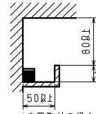
&lt;床置取付の場合&gt;
