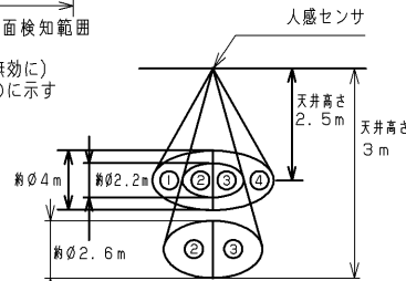
図D 検知範囲限定(無効)箇所
