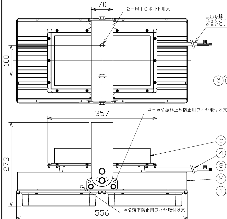
器具取付けボルトを使用した場合の器具内寸法 ※A寸法は、40mm以下にしてください。
