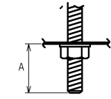
取付ボルトを使用した場合の器具内寸法
