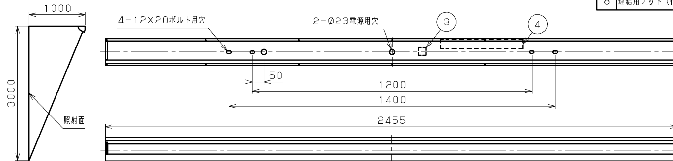
標準取付位置
