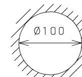
埋込み寸法 取付け可能天井厚: 5mm~25mm
