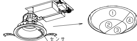
図D エリアカットシール（取扱説明書最終頁に添付）および貼り付け位置
