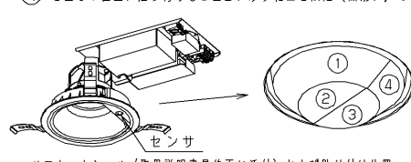
図D エリアカットシール（取扱説明書最終頁に添付）および貼り付け位置
