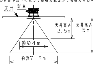
図A 天井から床面への検知範囲
