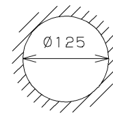
埋込み穴寸法 取り付け可能天井厚: 5mm~25mm
