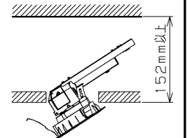
器具取り付け必要高さ
