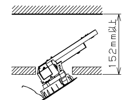
器具取付け必要高さ
