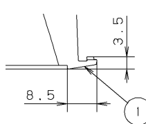
各部詳細
