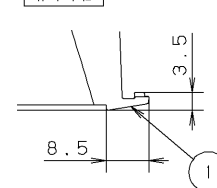
種部詳細
