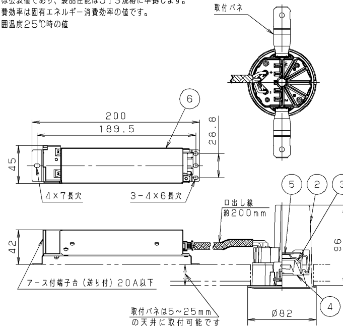
種部詳細
