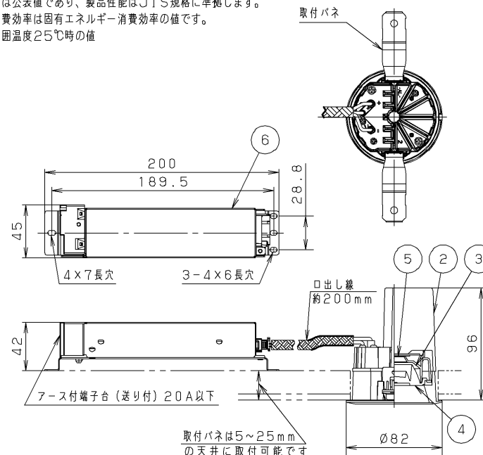
枠部詳細
