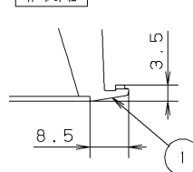
枠部詳細
