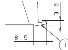
枠部詳細
