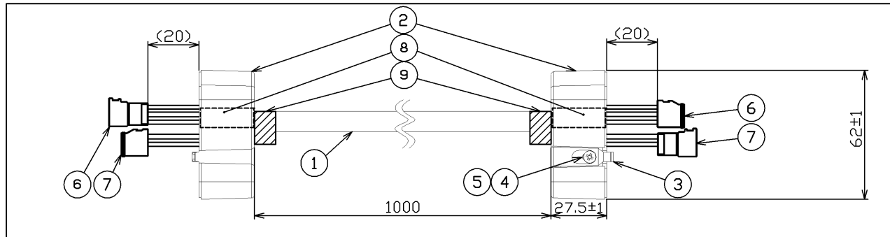
延長ケーブル LEB-L10013
