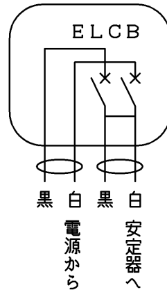
結線図
