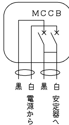
結線図
